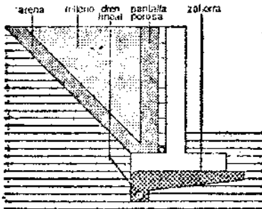
Sección vertical
