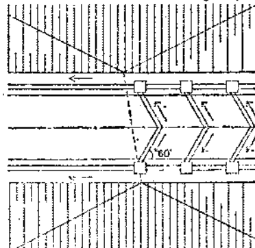
Planta Paso de desmonte a terrapién
