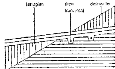
Sección longitudinal
